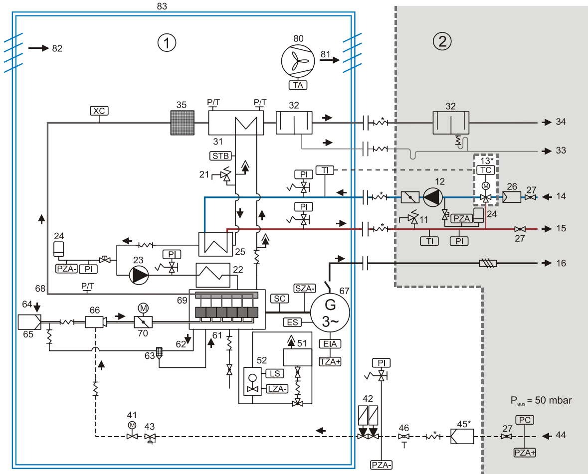
Рис. 2 Устройства контроля
