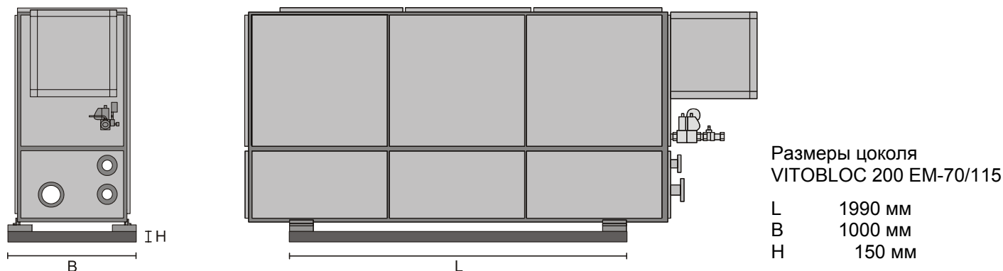
Рис. 7 Размер цоколя
